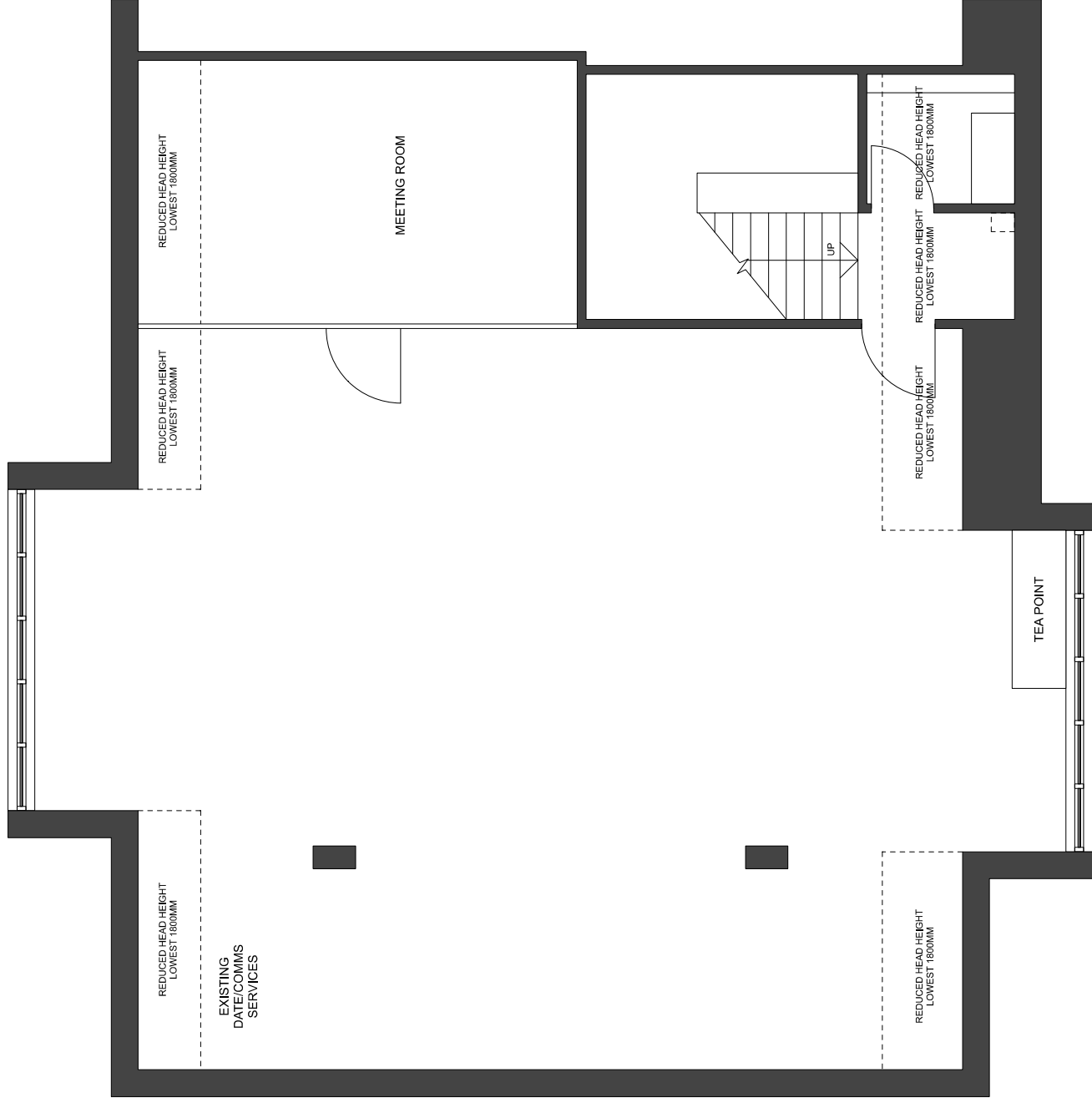
1 EXISTING FLOORPLAN Scale: 1:50
